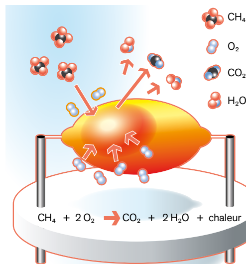
Figure 2 : Schéma de principe de fonctionnement d'un détecteur catalytique
