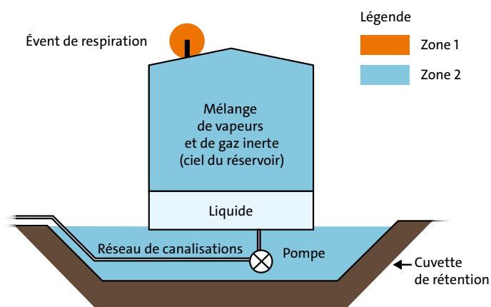
Figure n°8 : Représentation des zones Atex dans le cas d'un réservoir de stockage d'un liquide combustible stocké à une température supérieure à son point d'éclair et des équipements associés (cas d'un réservoir inerté).
