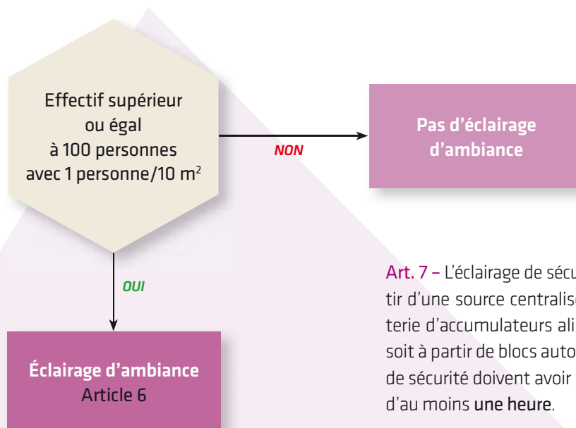
Fig. 7. Éclairage d'ambiance ou anti-panique
