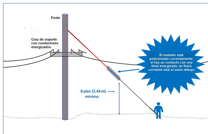
Figura 2. Ilustra la posición del aislador del cable de sujeción para evitar la electrificación del suelo.
