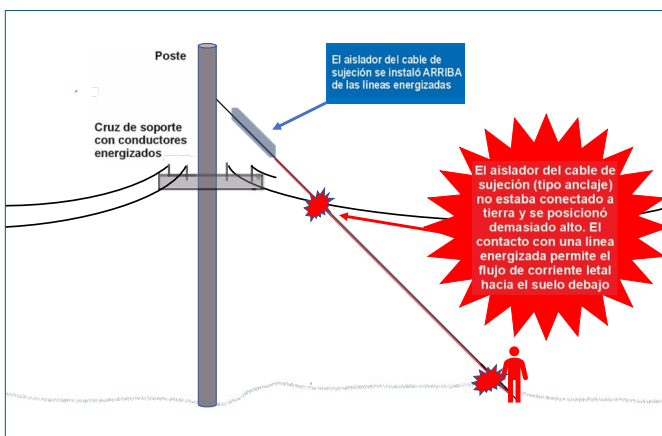
Figura 1. Ilustra cómo la colocación incorrecta de aisladores en el cable de sujeción puede crear un peligro significativo.
